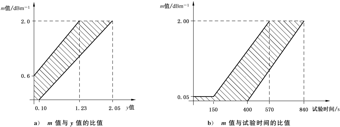
图 F.2 试验火合格判据
