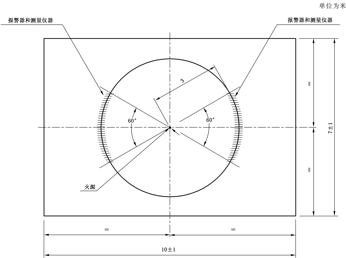
图 E.1 试验布置图
