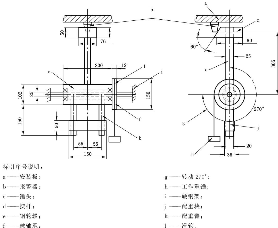
图 J.1 碰撞试验设备图
